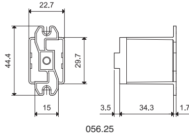
фланцевый адаптер крепления для реле 56.32
