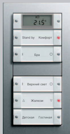
Gira E2 Сенсорный выключатель 2плюс, пятиклавишный цвет: "под алюминий" Новинка: с прозрачными клавишами
